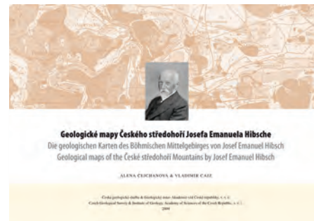
Alena Čejchanová, Vladimír Cajz: Geologické mapy Českého středohoří Josefa Emanuela Hibschke 467,-
