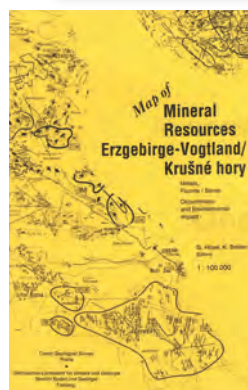
Map of Mineral Resources Erzgebirge-Vogtland/ Krušné hory a vysvětlivky, 1 : 100 000, slož. 436,-
