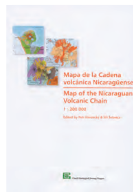
Mapa de la Cadena volcánica Nicaraguense/Map of the Nicaraguan Volcanic Chain, 1 : 200 000, slož. v obálce 363,-
